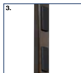
3. Predisposta per applicare una maniglia preesistente (es. portefinestre) e/o per un cilindro passante di una serratura con interasse 70 - 72 - 78 - 85 - 90 - 92 mm., (predisposizione dell'interasse regolabile).
